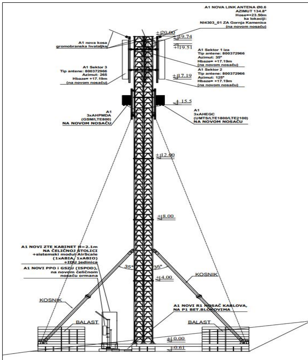
Слика 1.2. Планирана опрема будуће РБС
